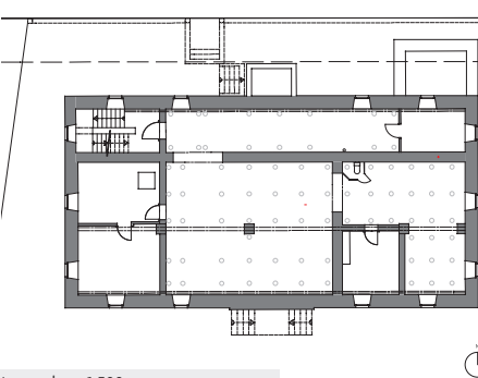
Untergeschoss 1:500
