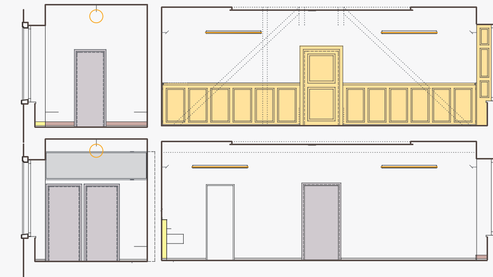
Abwicklung innen 1:100
